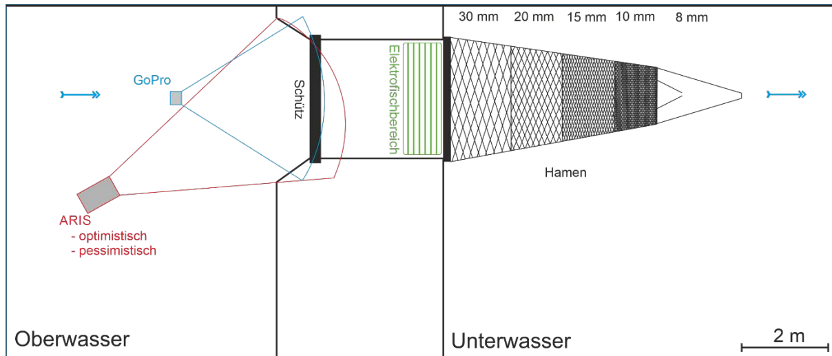
Abb. 1: Übersicht über den Versuchsaufbau aus der Vogelperspektive. Rot: Sonargerät, Blau: GoPro Kamera, Grün: Bereich der Elektrofishung. Mm-Angaben bezeichnen die sich verjüngenden Netzmaschenweiten des Hamens. Blaue Pfeile = Strömungsrichtung
