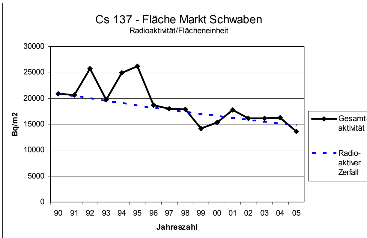
Abb. 9: Radioaktivitätsmesswerte (Cs 137) bis 30 cm Bodentiefe auf der Fläche Markt Schwaben zwischen 1990 und 2005
