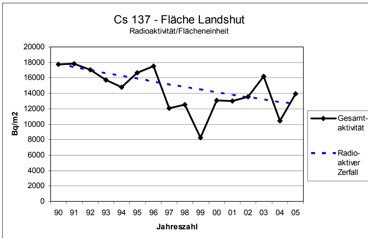
Abb. 6: Radioaktivitätsmesswerte (Cs 137) bis 30 cm Bodentiefe auf der Fläche Landshut zwischen 1990 und 2005
