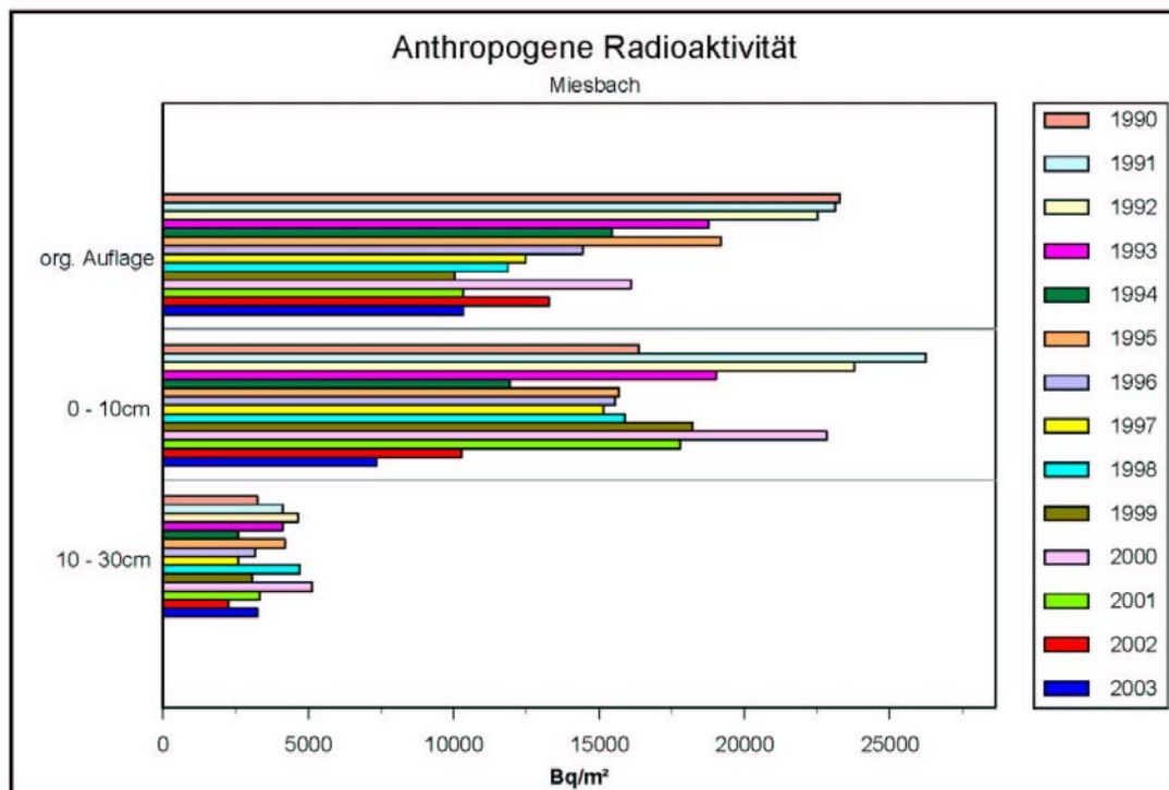
Abb. 13: Vertikale Verteilung der anthropogen induzierten Radioaktivität (Summe Cs 137, Cs 134, Sb 125, Ru 106, Ce 144) im Boden am Beispiel Miesbach
