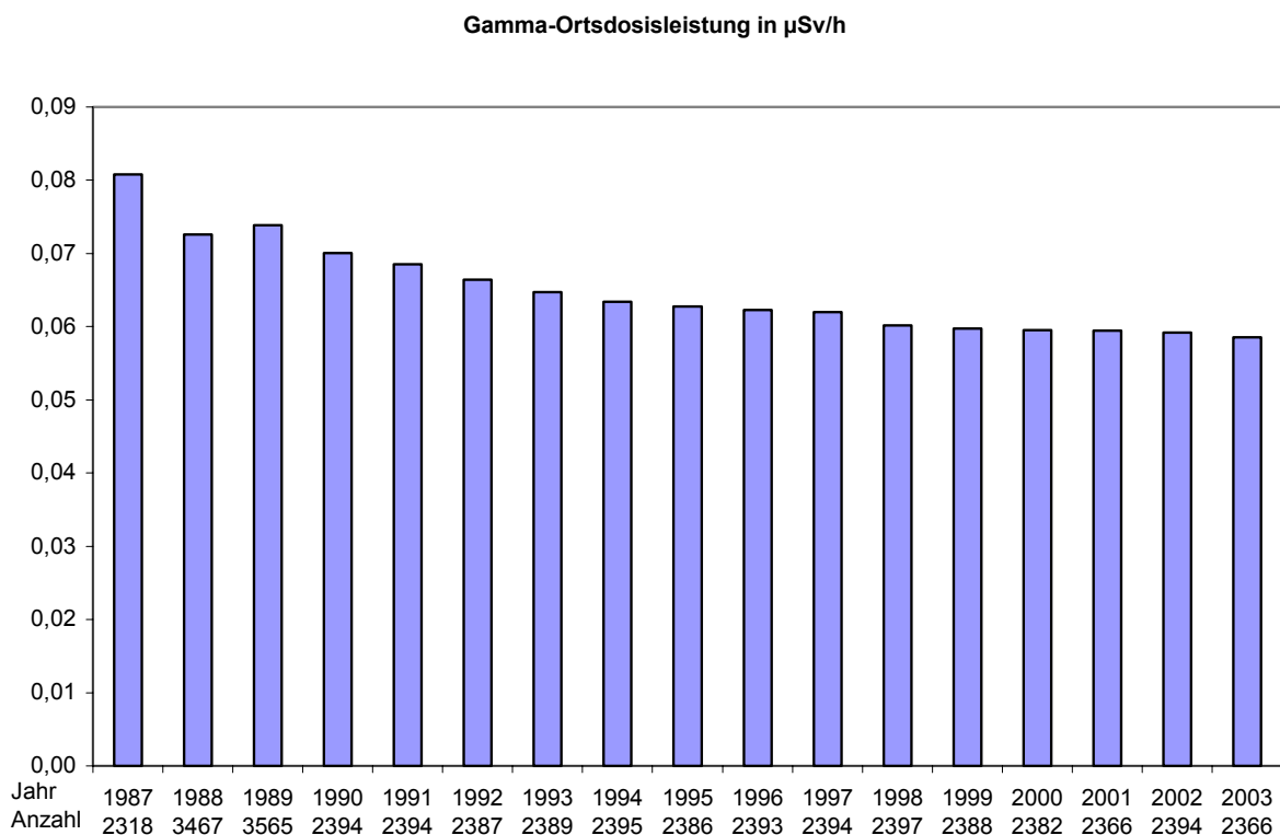
Abb. 11: Zeitverlauf der Abnahme der bayernweiten durchschnittlichen Gamma-Ortsdosisleistung in Mikrosievert pro Stunde von 1987 bis 2003. Die untere Abszissenachse gibt die Anzahl der jeweils vorgenommenen Messungen wieder.
