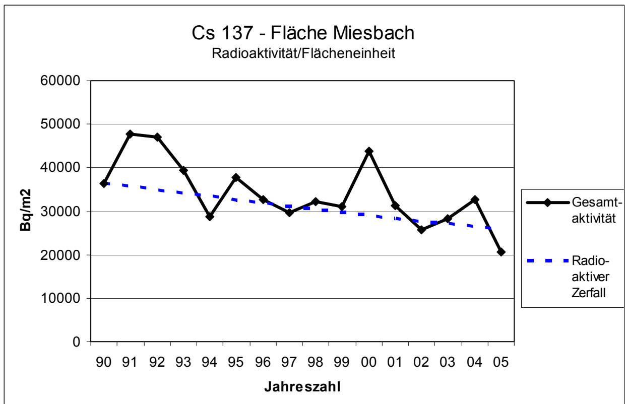
Abb. 12: Radioaktivitätsmesswerte (Cs 137) bis 30 cm Bodentiefe auf der Fläche Miesbach zwischen 1990 und 2005
