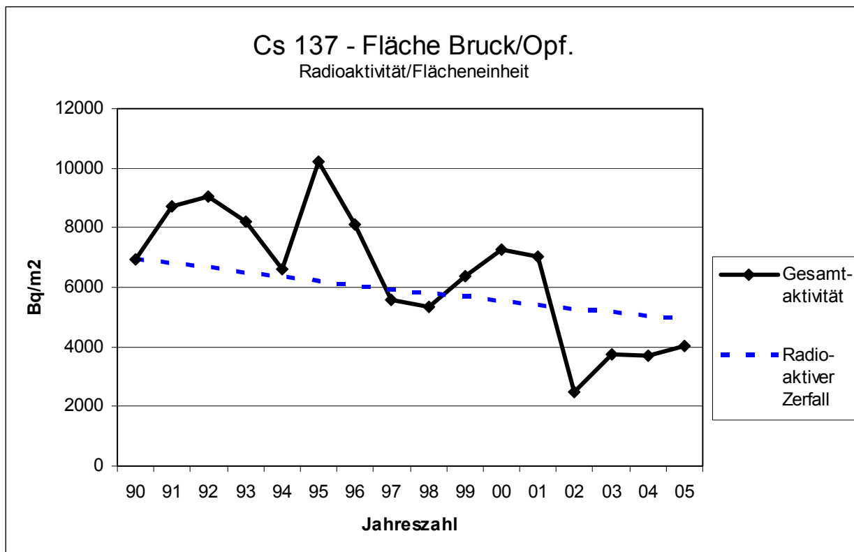
Abb. 5: Radioaktivitätsmesswerte (Cs 137) bis 30 cm Bodentiefe auf der Fläche Bruck/Opf. zwischen 1990 und 2005
