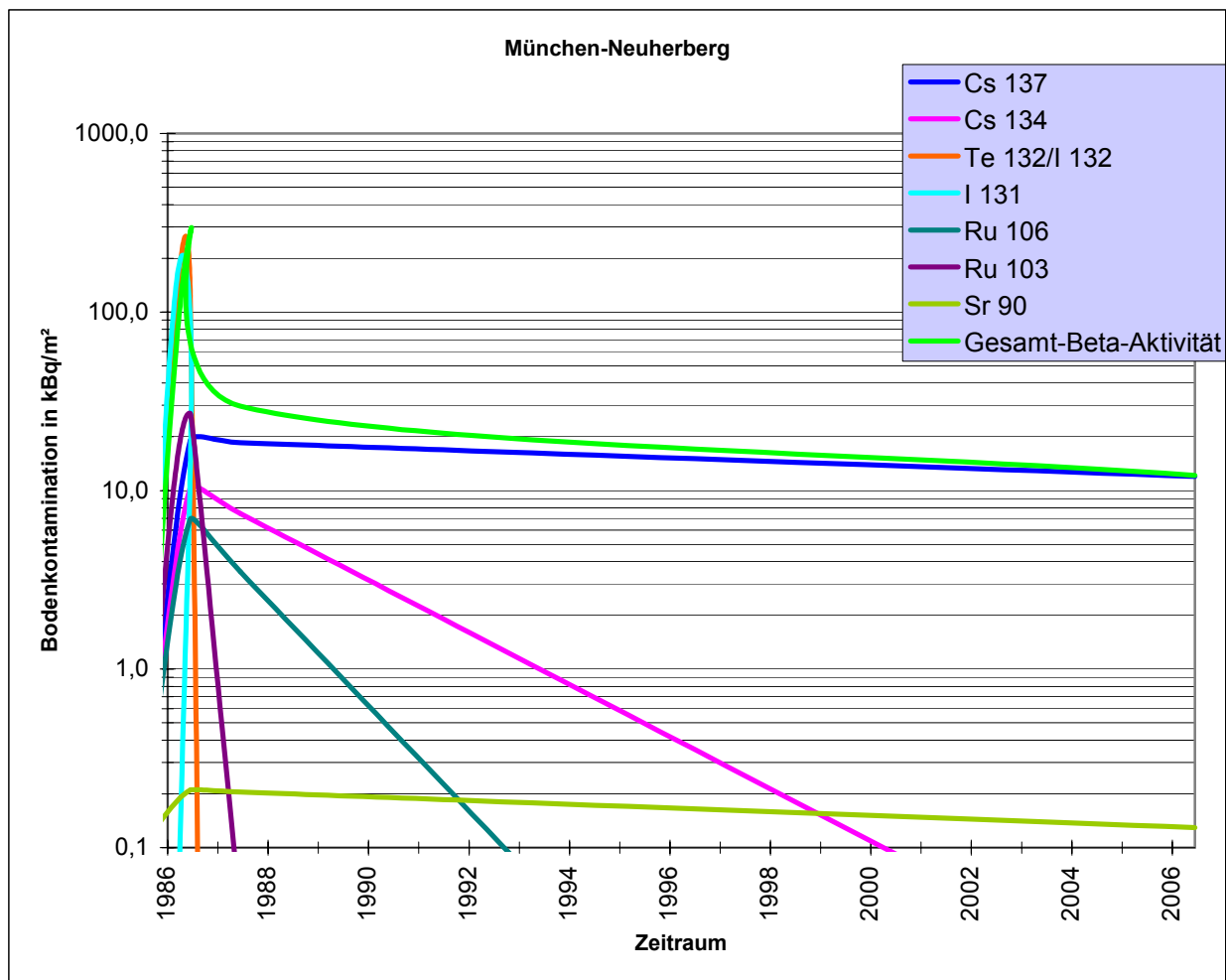
Abb. 10: Abklingkurven der aus dem natürlichen radioaktiven Zerfall zu erwartenden zeitlichen Veränderungen der seinerzeit in München-Neuherberg festgestellten Bodenkontamination.
