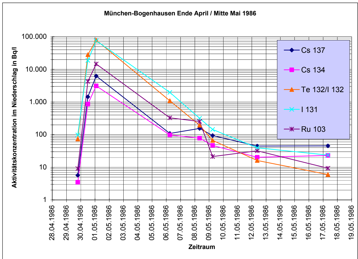
Abb. 7: Zeitverlauf der Aktivitätskonzentration im Niederschlag von München-Bogenhausen, gemessen vom Bayerischen Landesamt für Umwelt (LfU).
