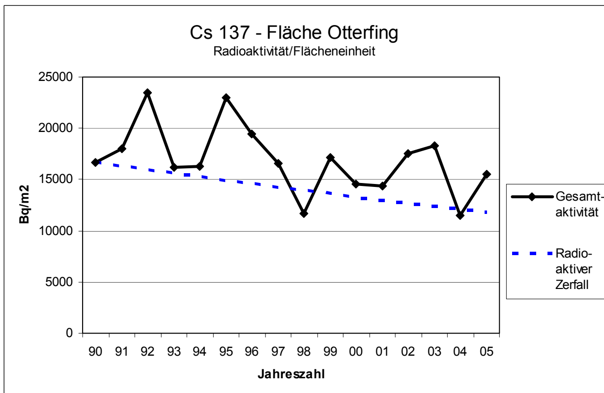
Abb. 10: Radioaktivitätsmesswerte (Cs 137) bis 30 cm Bodentiefe auf der Fläche Otterfing zwischen 1990 und 2005
