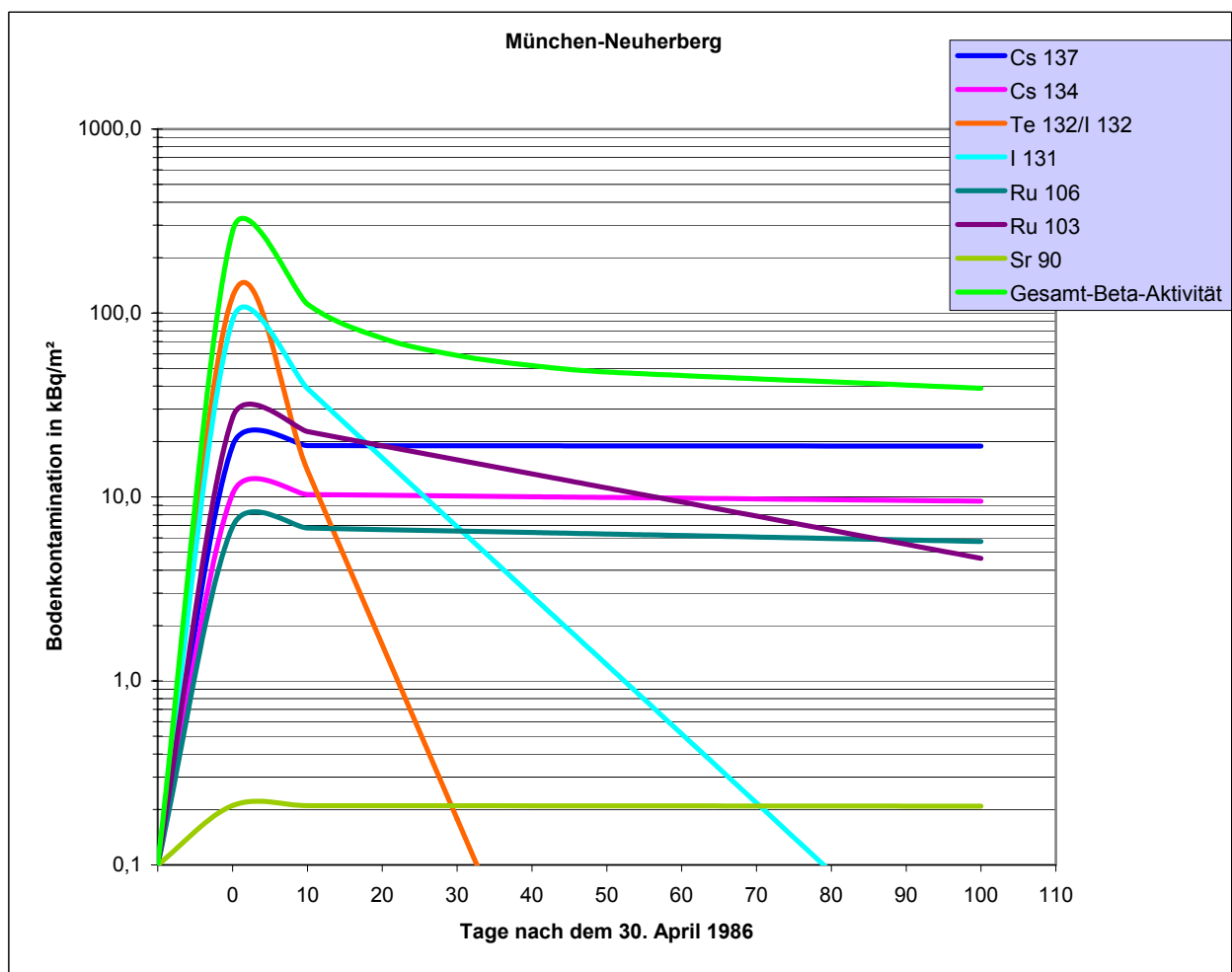
Abb. 9: Nuklidzusammensetzung der abgelagerten Aktivität auf dem Boden in München-Neuherberg und deren zu erwartende zeitliche Änderung infolge radioaktiven Zerfalls, gemessen vom Forschungszentrum für Umwelt und Gesundheit GSF.
