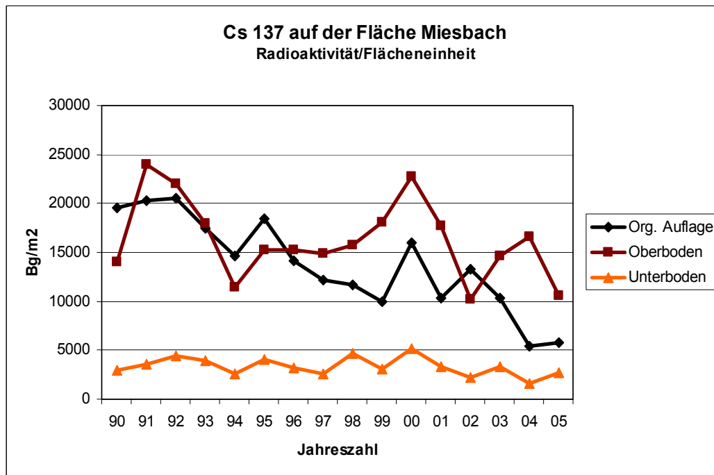
Abb. 15: Verlauf der Radioaktivitäten (Cs 137) in Abhängigkeit von den Bodentiefen auf der Fläche Miesbach
