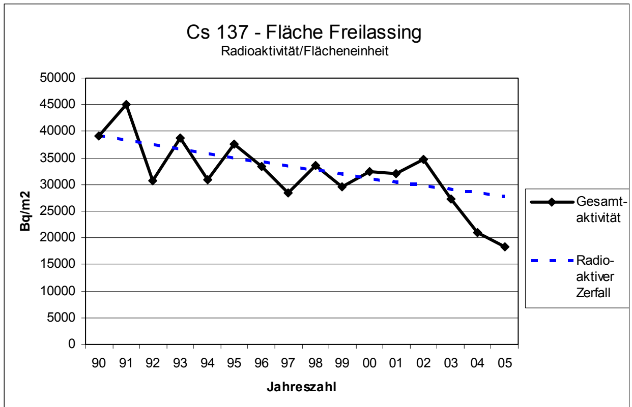
Abb. 11: Radioaktivitätsmesswerte (Cs 137) bis 30 cm Bodentiefe auf der Fläche Freilassing zwischen 1990 und 2005
