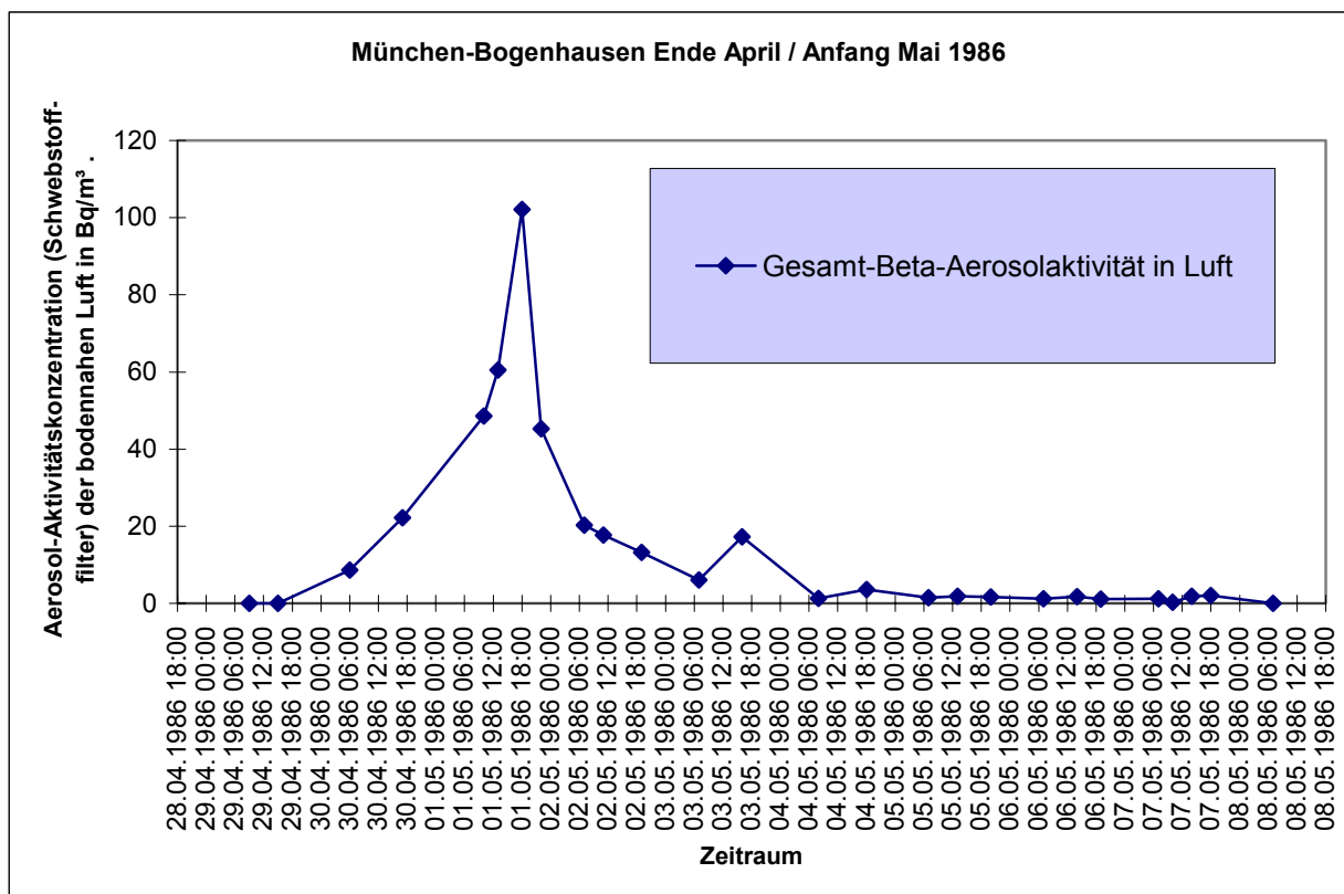
Abb. 6: Zeitverlauf der Gesamt-Beta-Aktivität in der bodennahen Luft in München-Bogenhausen während des Durchzugs der Wolke, ermittelt vom Bayerischen Landesamt für Umwelt (LfU).
