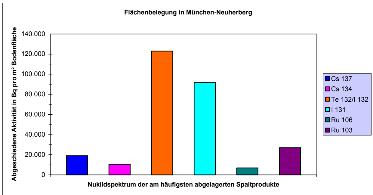
Abb. 8: Nuklidspezifische Flächenbelegung infolge des Tschernobyl-Unfalls in München-Neuherberg, ermittelt vom Forschungszentrum für Umwelt und Gesundheit GSF [6].
