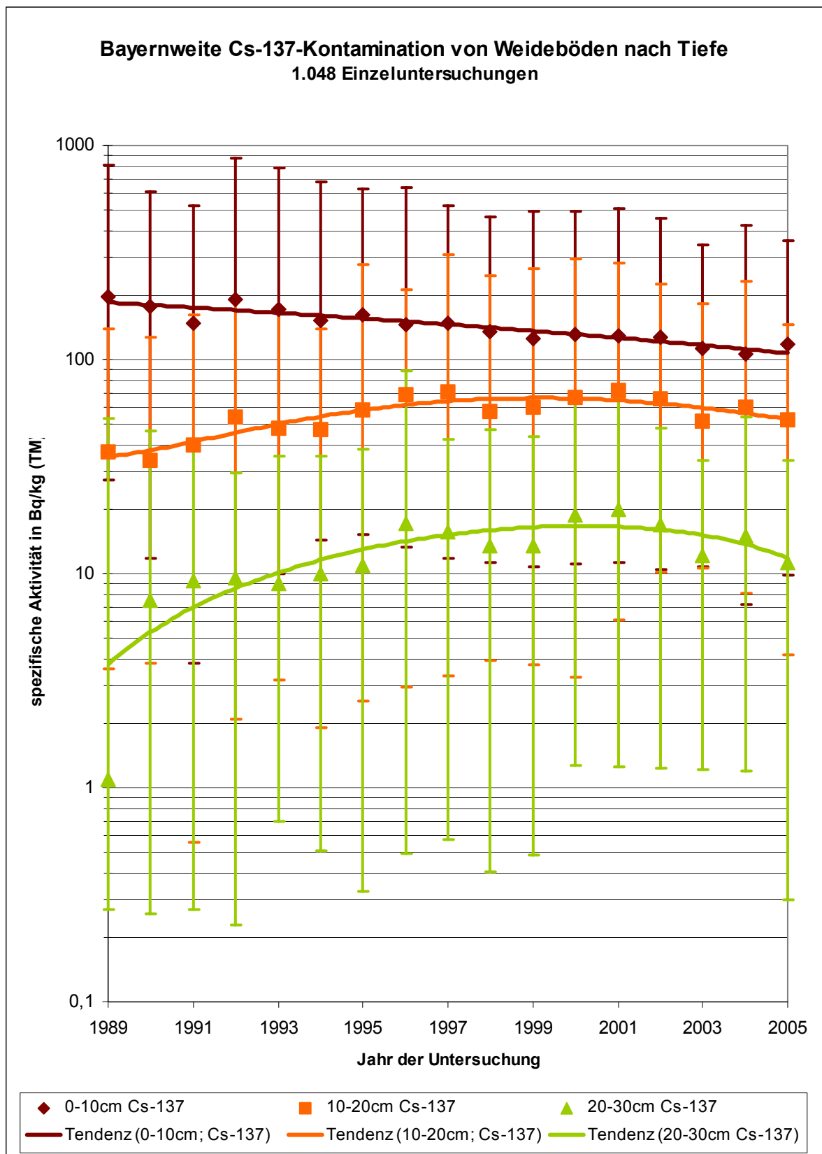
Abb. 22: Zeitverlauf der bayernweiten Cäsium-137-Kontamination von Weideböden in Tiefenabhängigkeit.
