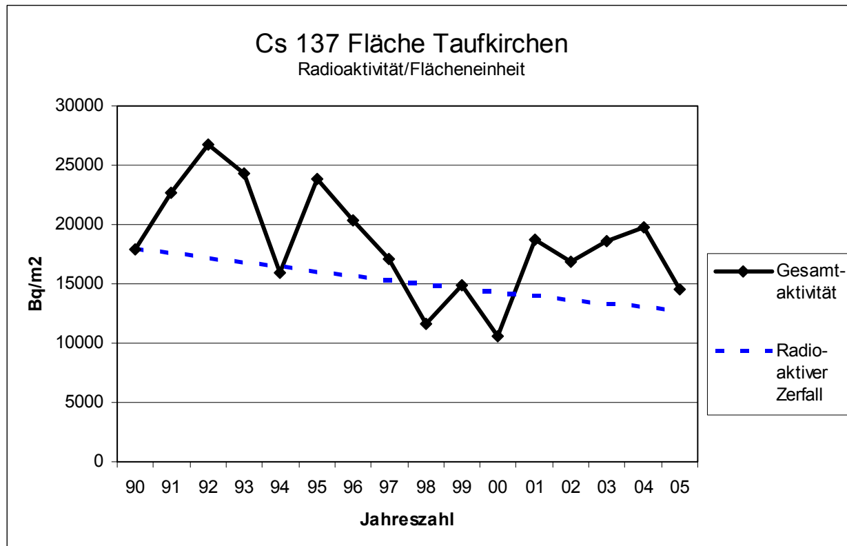
Abb. 7: Radioaktivitätsmesswerte (Cs 137) bis 30 cm Bodentiefe auf der Fläche Taufkirchen zwischen 1990 und 2005
