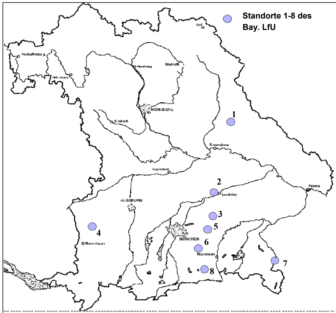
Abb. 1: Standorte der R-BDF, angelegt im Rahmen der Umsetzung des Strahlenschutzvorsorgegesetzes in Bayern
