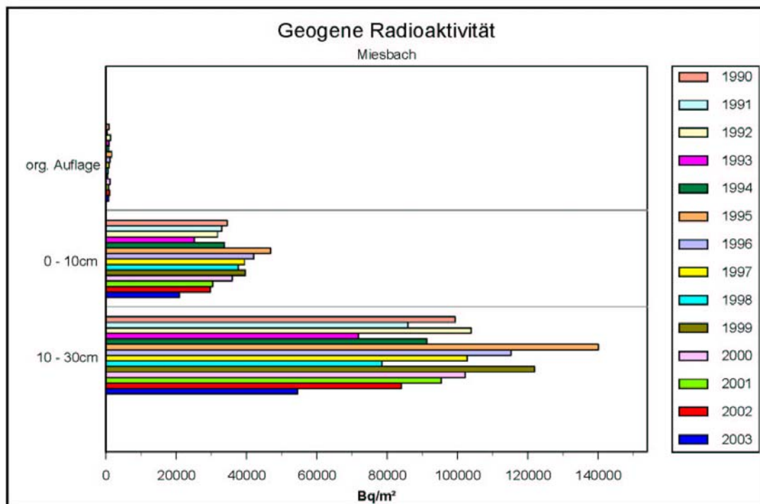
Abb. 14: Vertikale Verteilung der geogen vorhandenen Radioaktivität (Summe K 40, Ac 228, Ra 226) im Boden am Beispiel Miesbach
