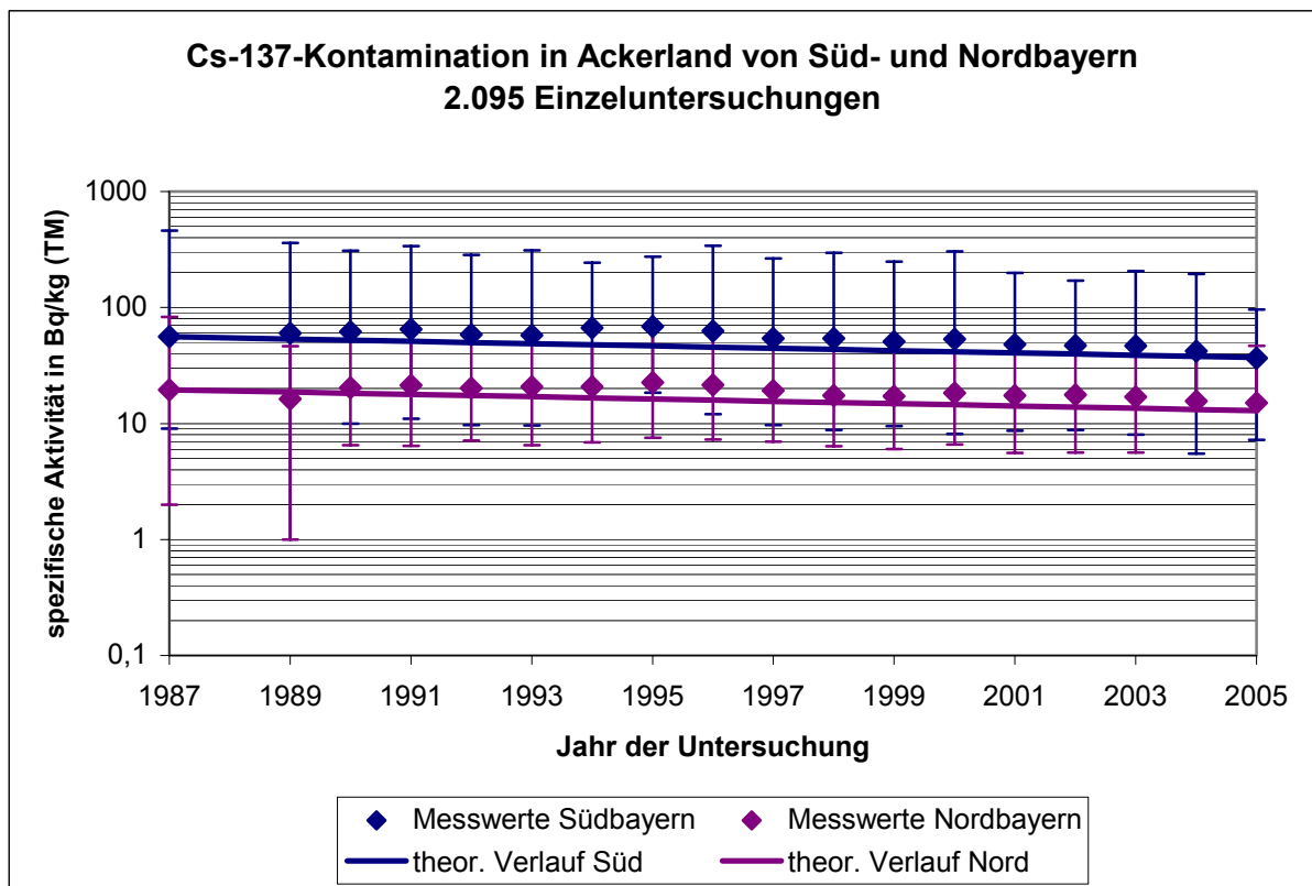
Abb. 16: Zeitverlauf der Cäsium-137-Kontamination von Ackerland.
