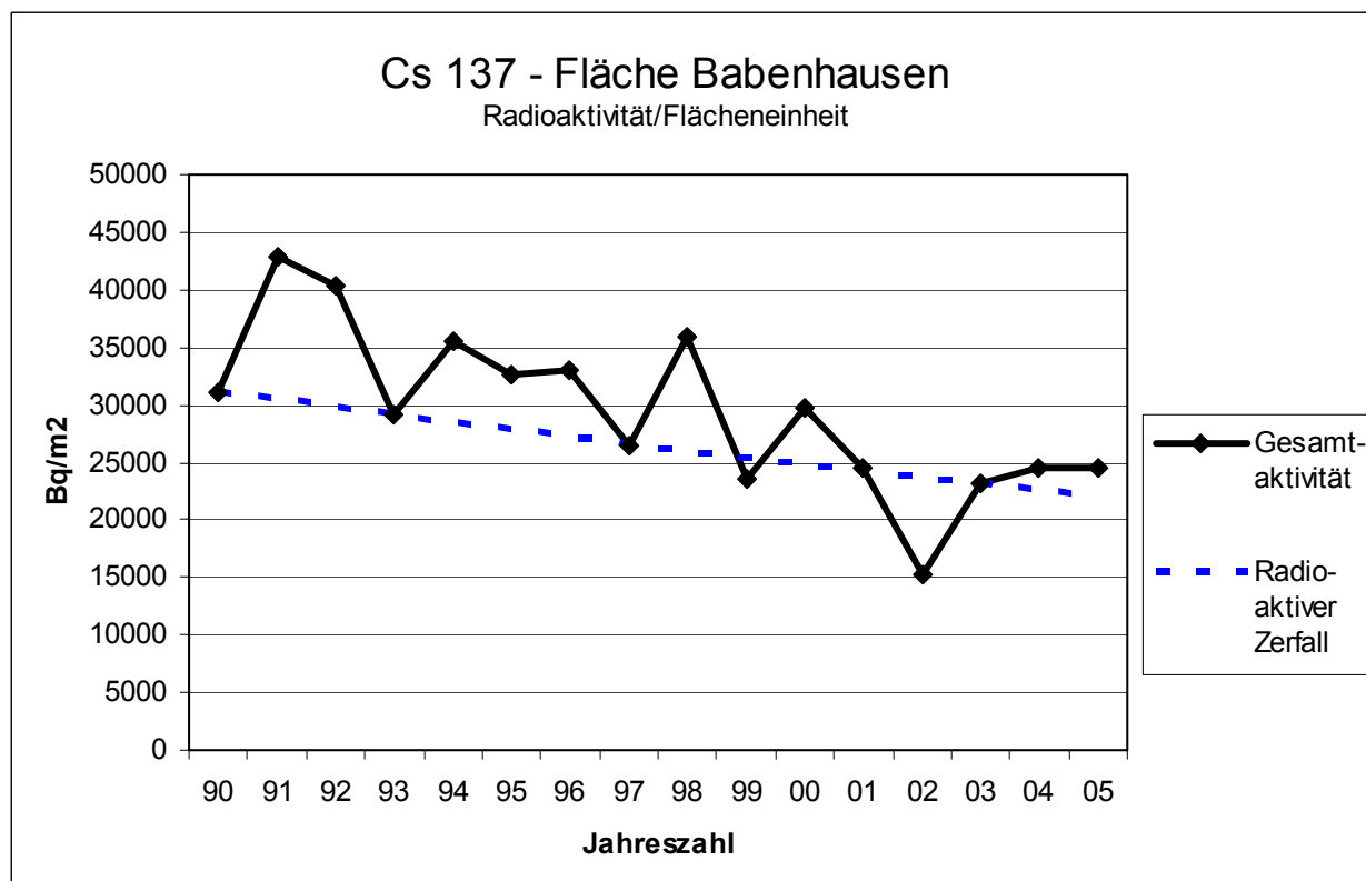
Abb. 8: Radioaktivitätsmesswerte (Cs 137) bis 30 cm Bodentiefe auf der Fläche Babenhausen zwischen 1990 und 2005
