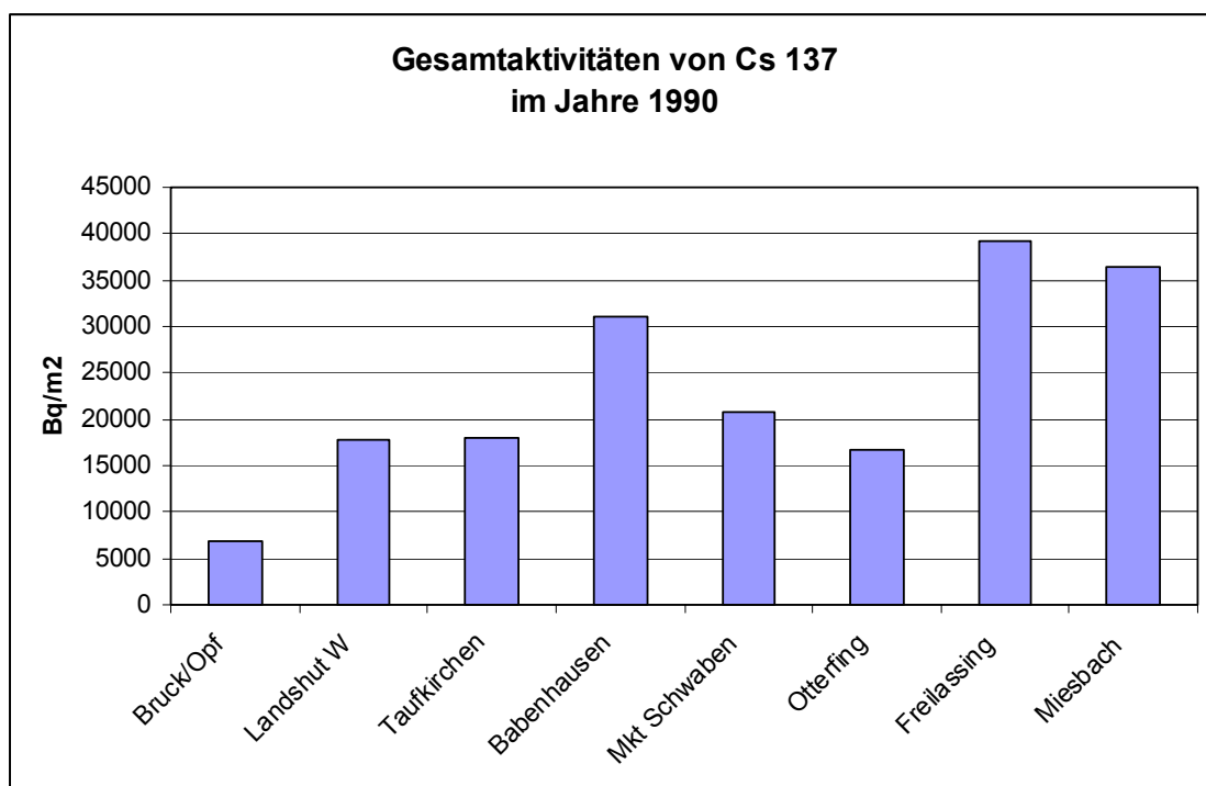
Abb. 4: Radioaktivitäten auf den 8 Messflächen bis 30 cm Bodentiefe im Vergleich (gemessen 1990)
