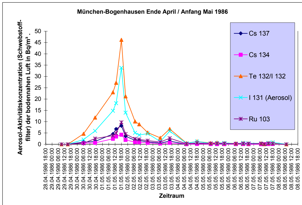
Abb. 5: Nuklidspezifische Aerosol-Aktivitätskonzentration in der bodennahen Umgebungsluft des Bayerischen Umweltministeriums in München-Bogenhausen während des Durchzugs der radioaktiven Wolke aus Tschernobyl, gemessen vom Bayerischen Landesamt für Umwelt (LfU).
