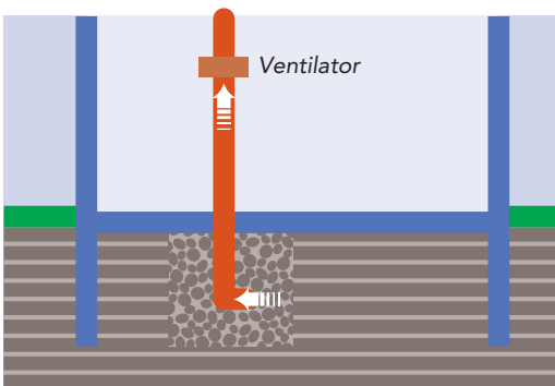
Punktueller Unterboden-Absaugung mit Abluft über Dach.
