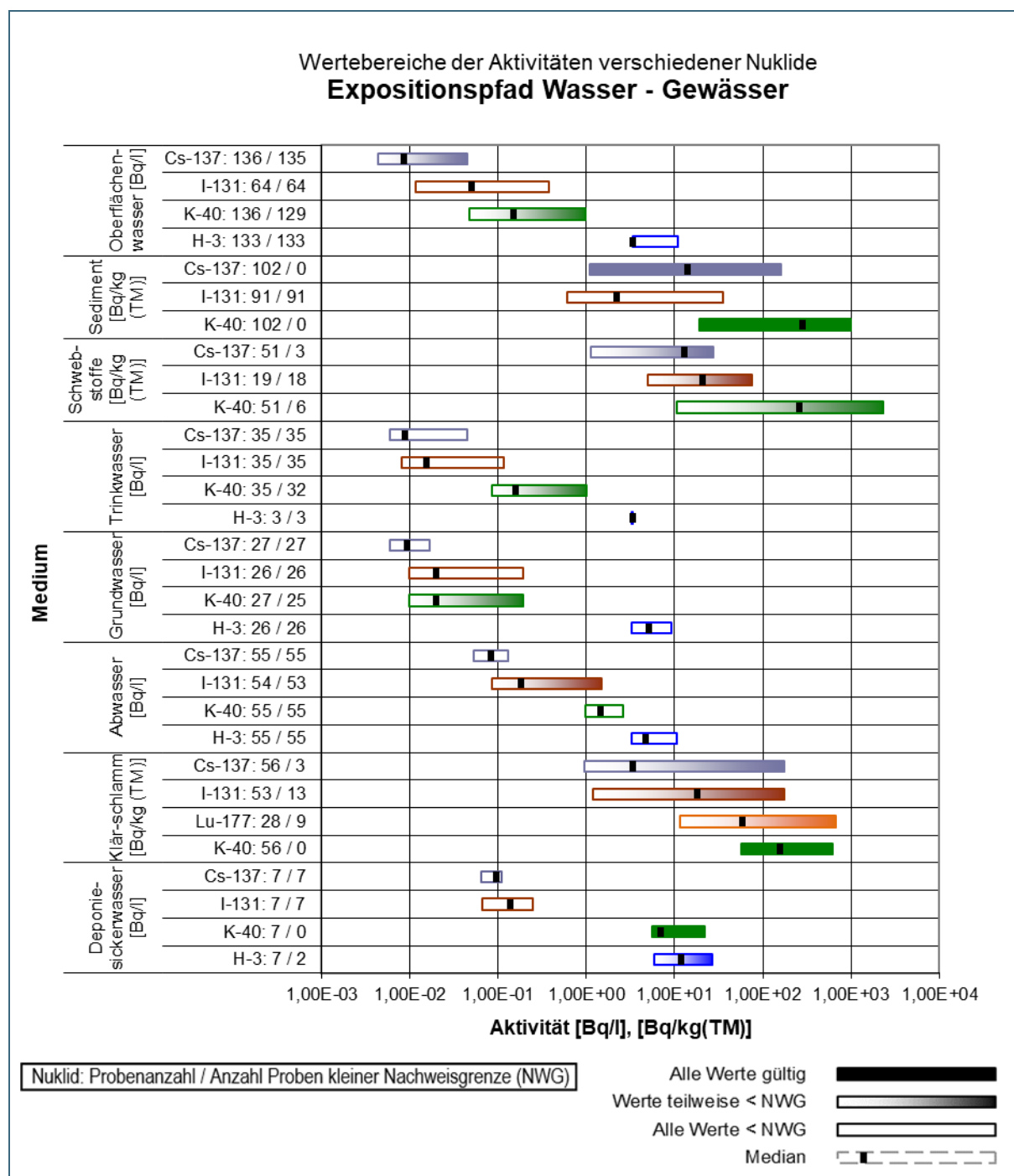
Abb. 2: Wertebereiche der in Bayern gemessenen Aktivitäten des Expositionspfad Wasser im Jahr 2024
