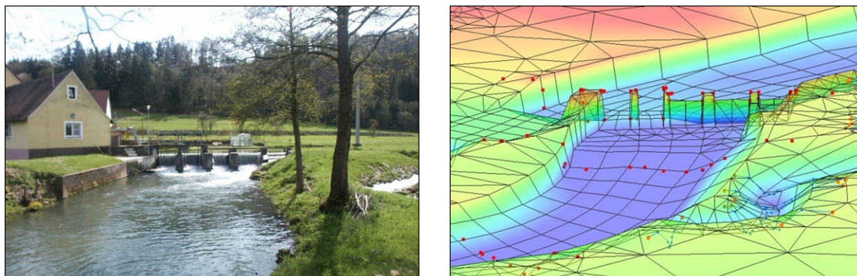
Foto und entsprechend nachgebildetes Modell eines Flusslaufs
