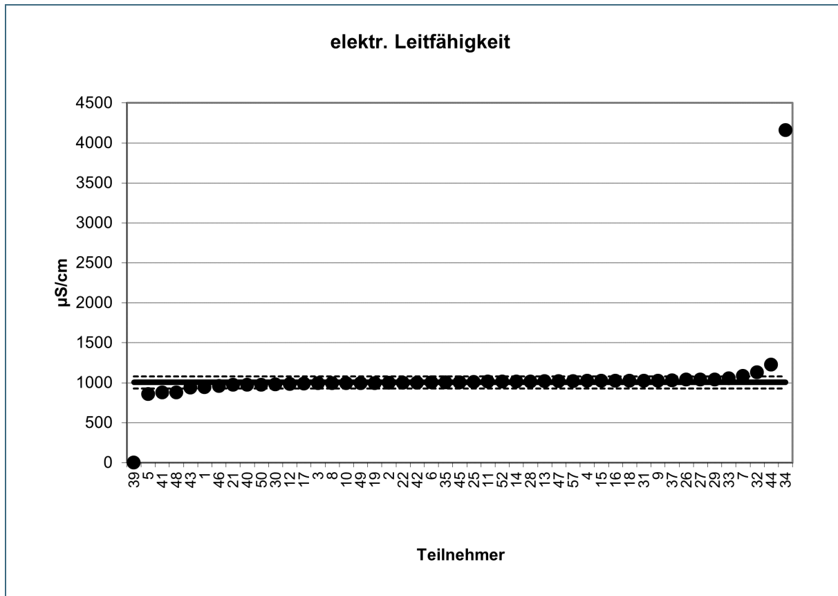
Abb. 33: Elektrische Leitfähigkeiten aller Teilnehmer mit Toleranzgrenzen
