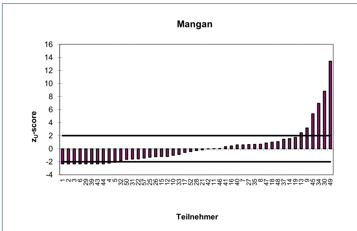
Abb. 82: Mangan – zU-Scores der Konzentrationen der Teilnehmer
