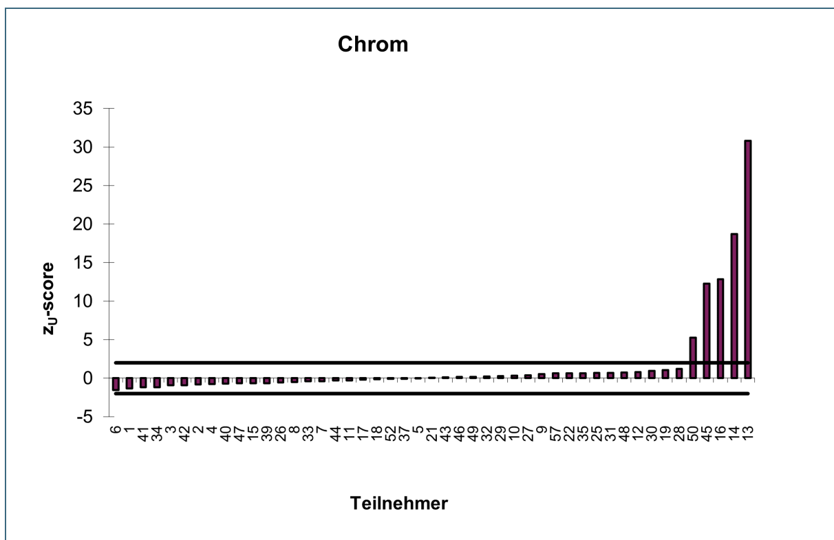
Abb. 70: Chrom – z U -Scores der Konzentrationen der Teilnehmer
