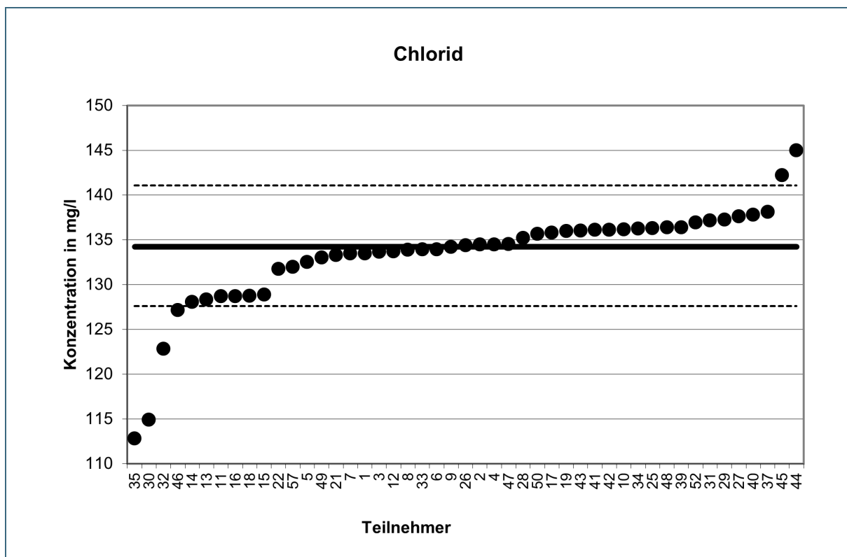
Abb. 55: Chlorid in mg/l – Konzentrationen aller Teilnehmer mit Toleranzgrenzen
