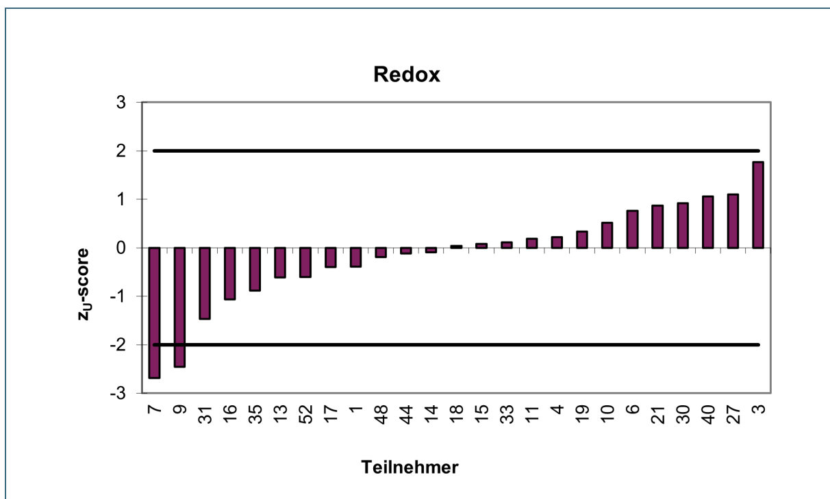
Abb. 39: Redoxpotential in mV H – Z U -Scores der Teilnehmer
