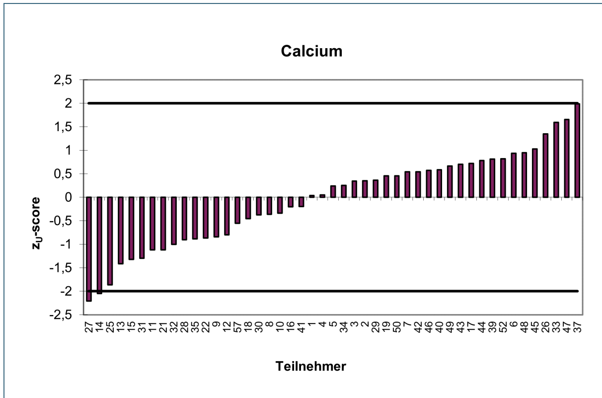
Abb. 43: Calcium – z U -Scores der Teilnehmer
