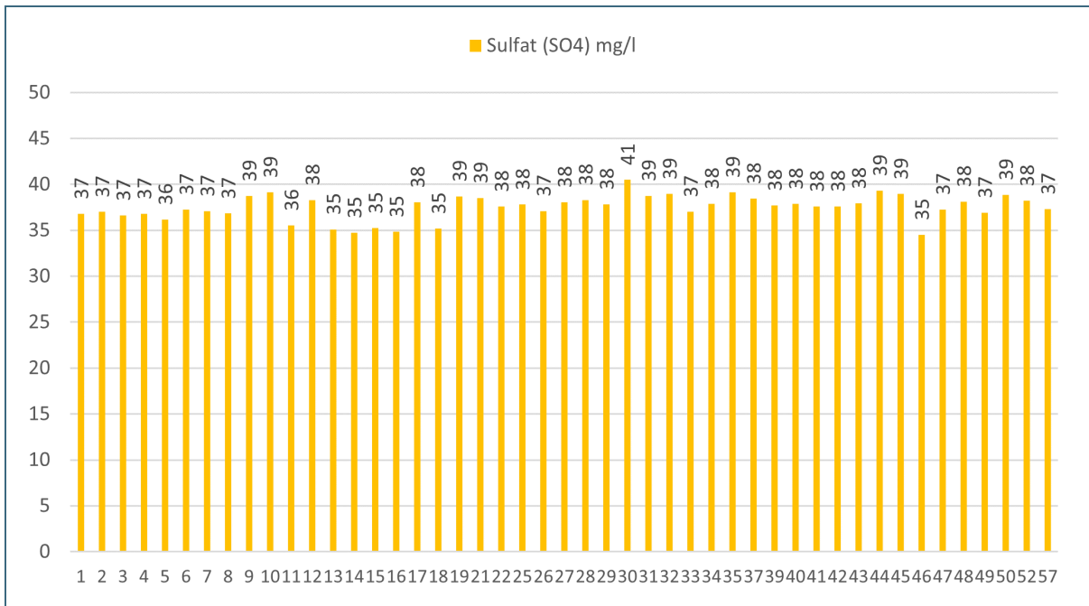
Abb. 60: Sulfat - Ergebnisse – Teilnehmer und Vergleichsprobennehmer
