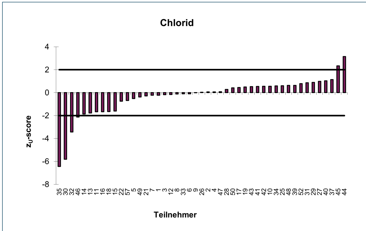
Abb. 56: Chlorid – z u -Scores der Teilnehmer
