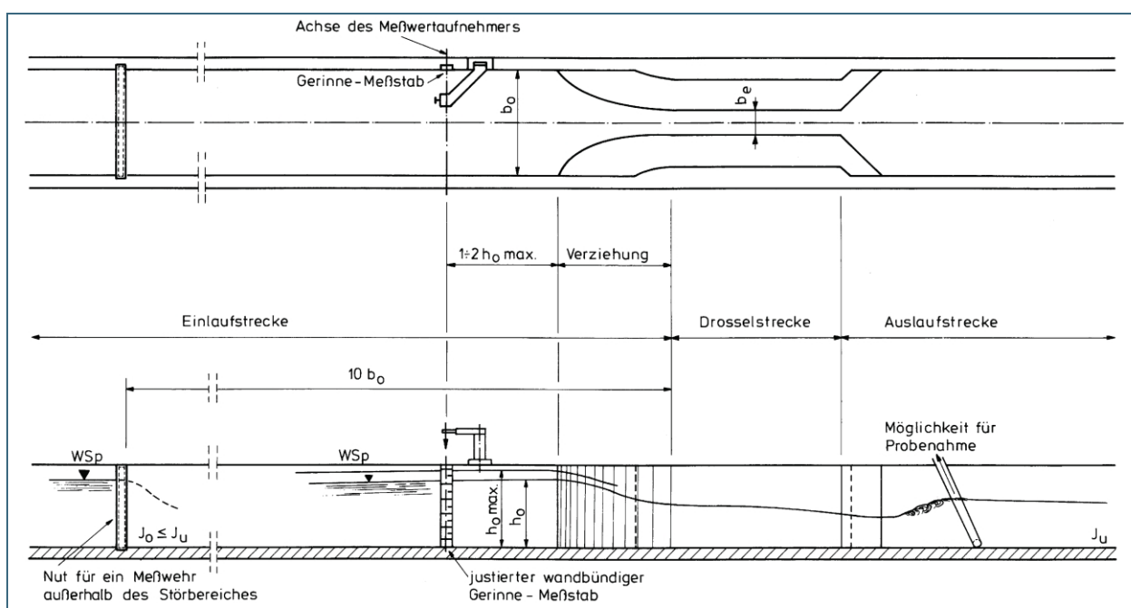
Abb. 5: Prinzipskizze eines Venturi-Gerintes ( h_0 =Oberwasserhöhe; b_0 =Gerinnebreite und b_e =Breite der Einengung)
