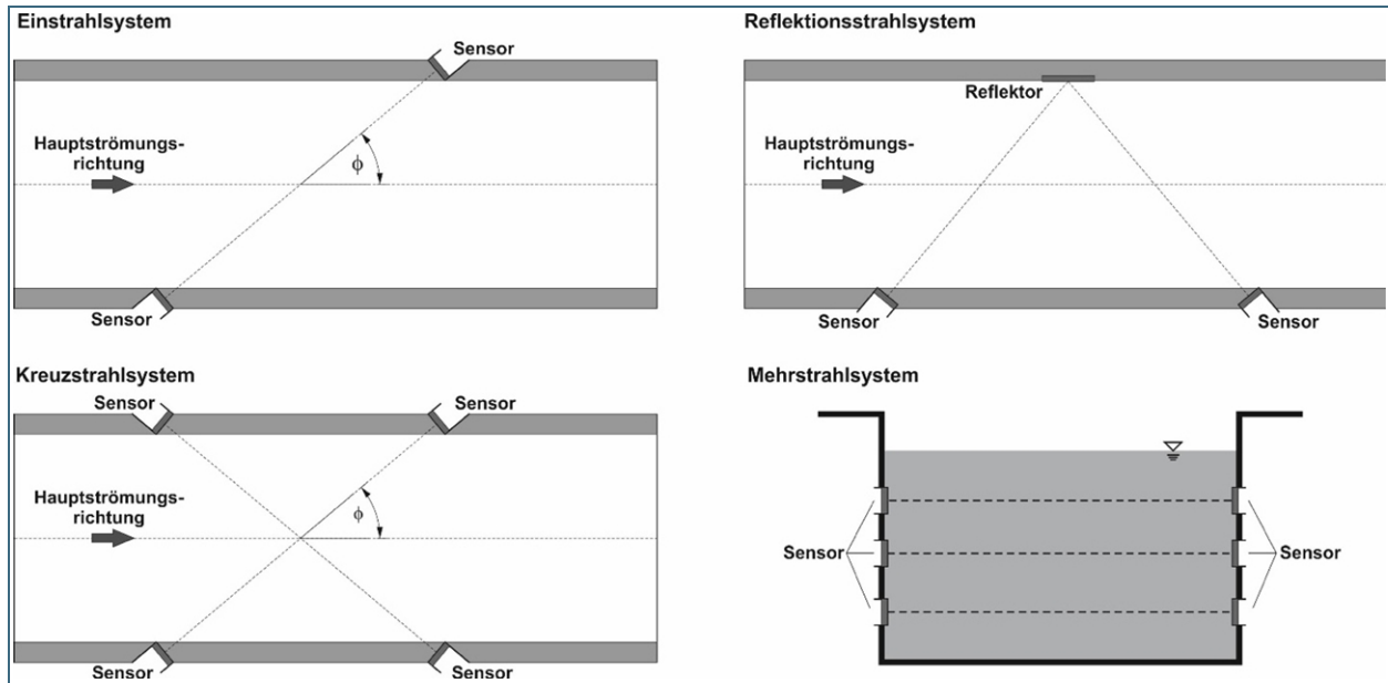
Abb. 8: Skizze eines Ultraschall-Laufzeitverfahrens und mögliche Anordnung von Messsensoren (Quelle: DWA Deutsche Vereinigung für Wasserwirtschaft, Abwasser und Abfall e. V.: Merkblatt DWA-M 181-2 „Messung von Wasserstand und Durchfluss in Entwässerungssystemen“, Dr. Ivo Baselt Universität der Bundeswehr München, 2023)
