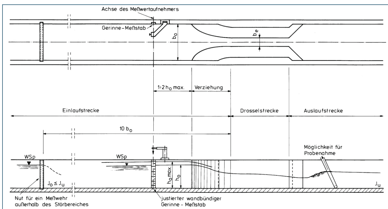
Abb. 5: Prinzipskizze eines Venturi-Gerinnes ( h_0 =Oberwasserhöhe; b_0 =Gerinnebreite und b_e =Breite der Einengung)
