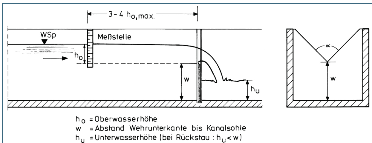
Abb. 1: Prinzipskizze eines Dreieck-Messwehrs
